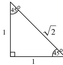
อัตราส่วนตรีโกณมิติของ มุม 45 องศา
