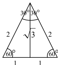
อัตราส่วนตรีโกณมิติของ มุม 30 และ 60 องศา
